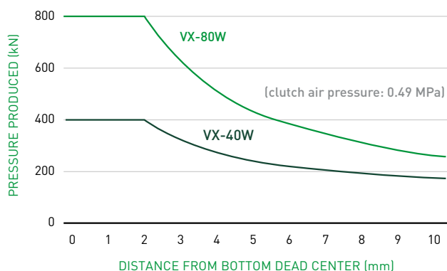
TONNAGE DIAGRAM
